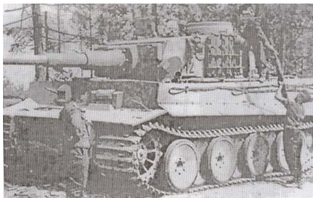
«Тигр» на широких гусеницах
